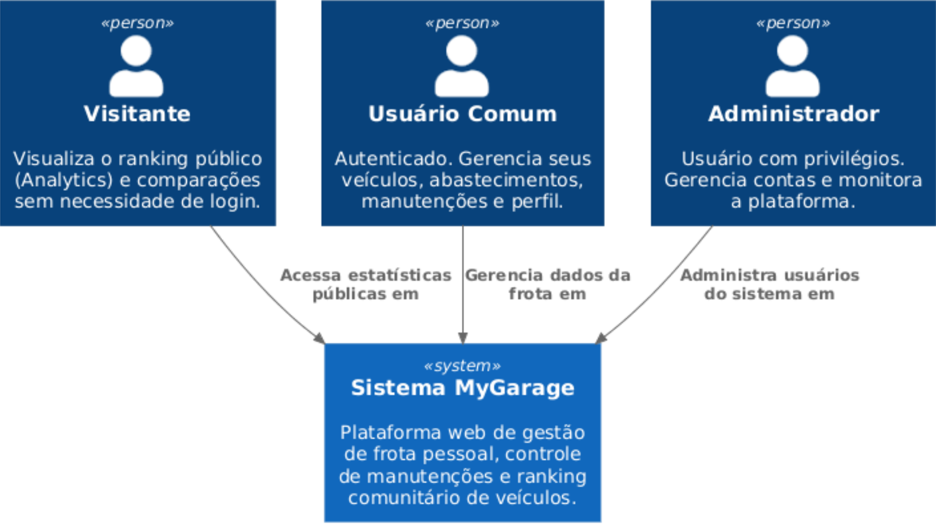
Diagrama de Contexto (C4 Nível 1) - Plataforma MyGarage
