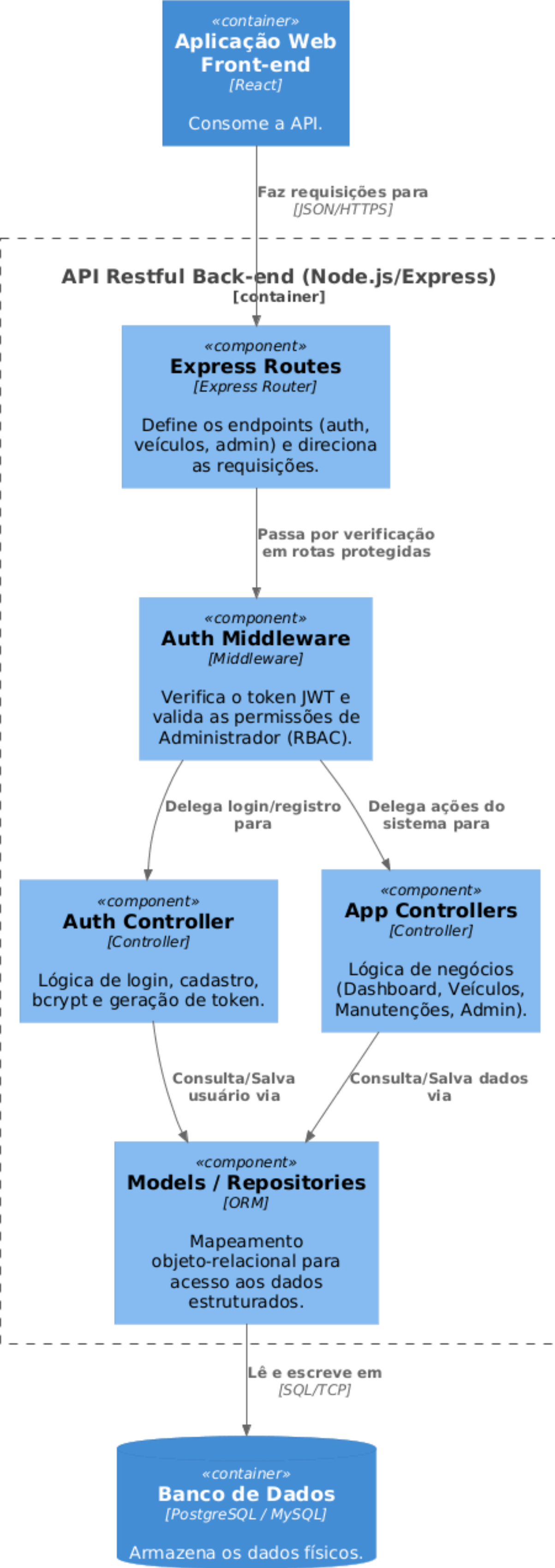
Diagrama de Componentes (C4 Nível 3) - Back-end API
