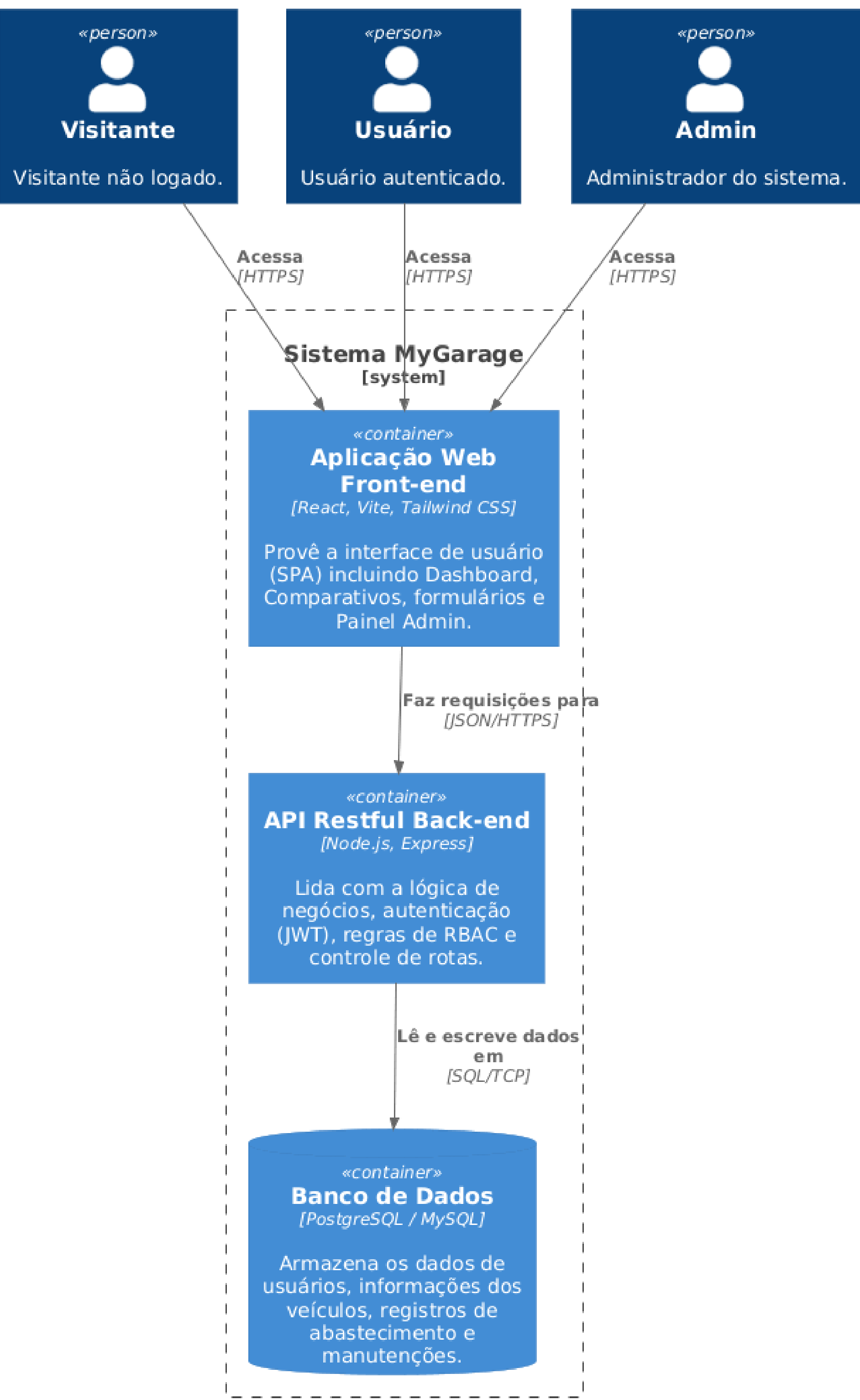
Diagrama de Container (C4 Nível 2) - Plataforma MyGarage
