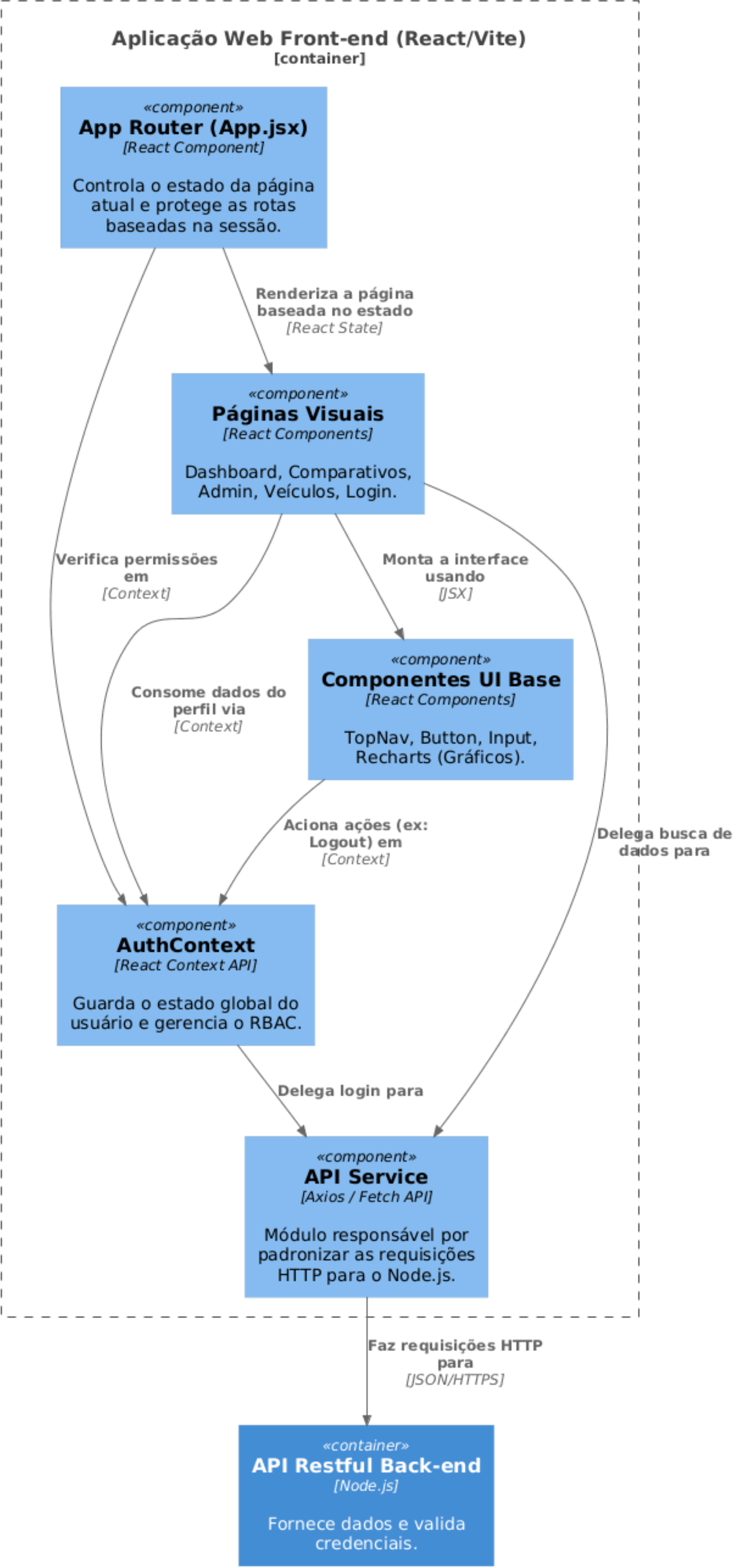
Diagrama de Componentes (C4 Nível 3) - Front-end
